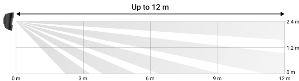
Poziomy kąt obserwacji czujnika
